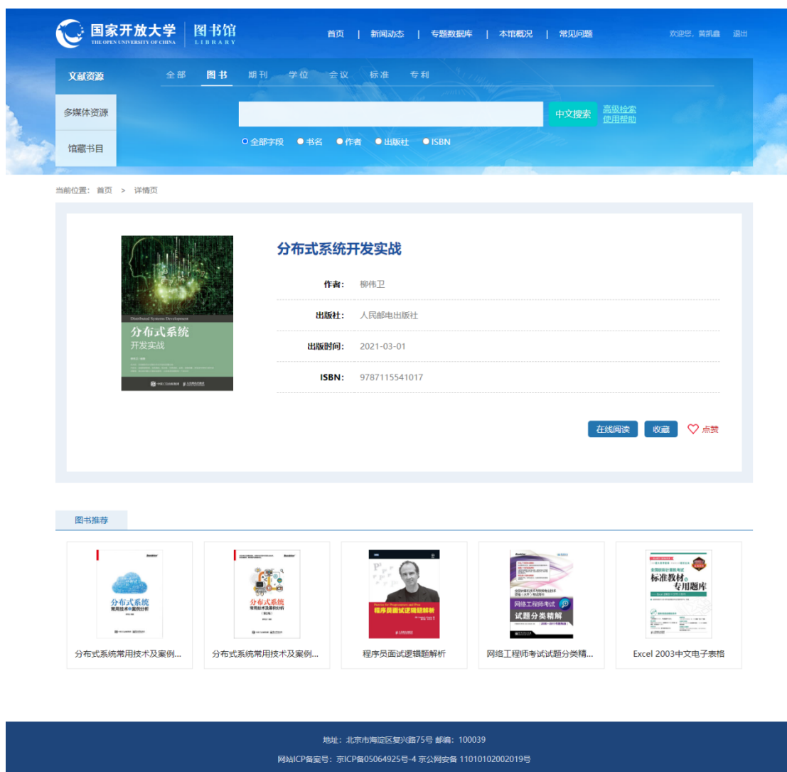
图 3-1-4 图书详情页
