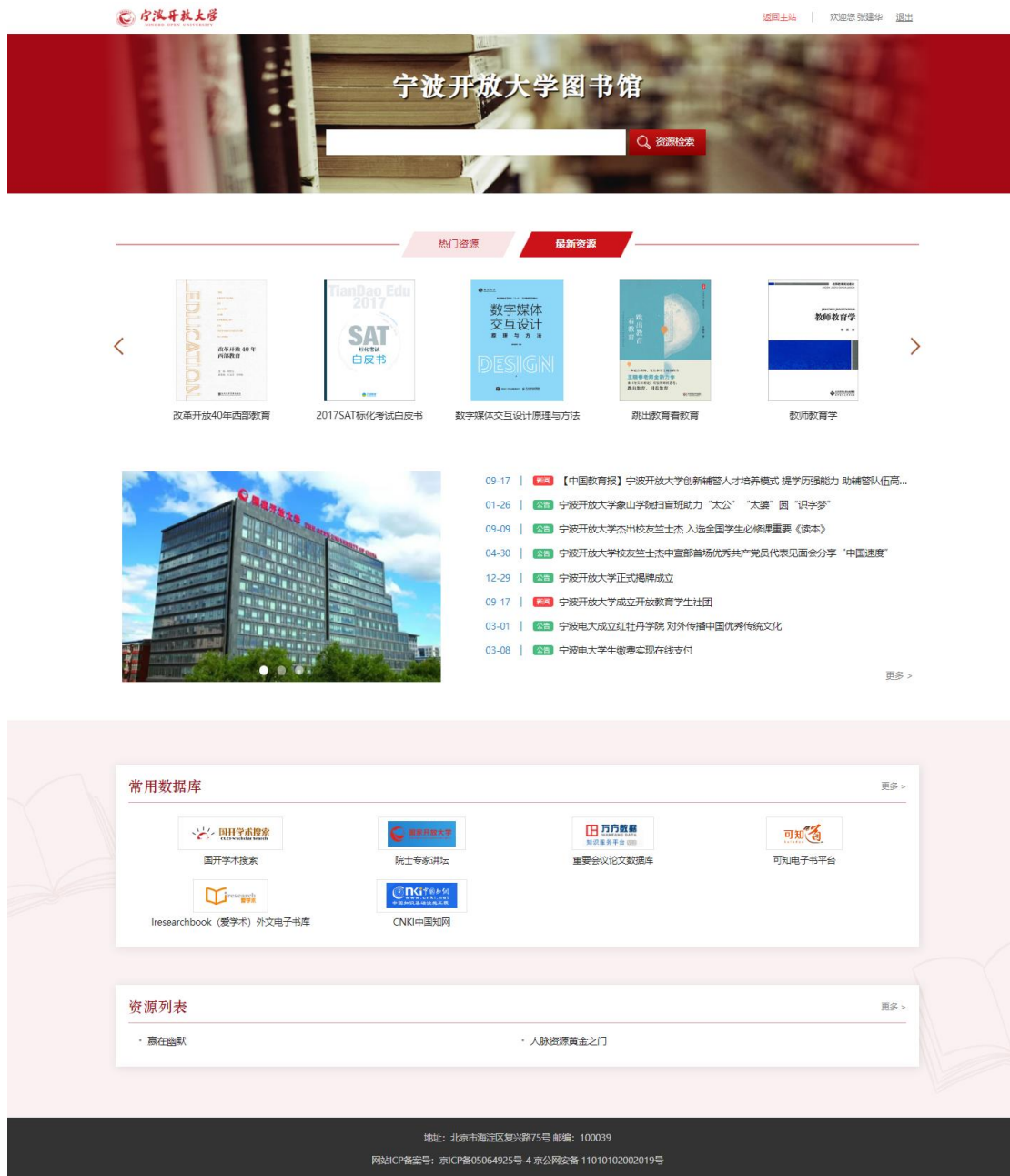
图 12-1 虚拟门户
