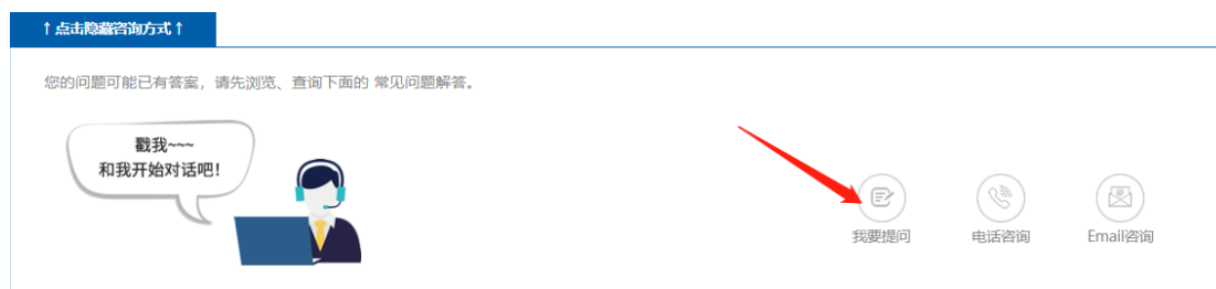
图 13-3-1 我要提问
